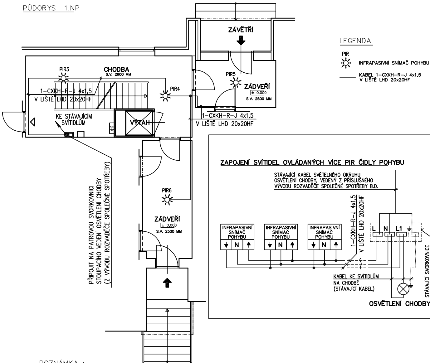
PŮDORYS 1.NP
