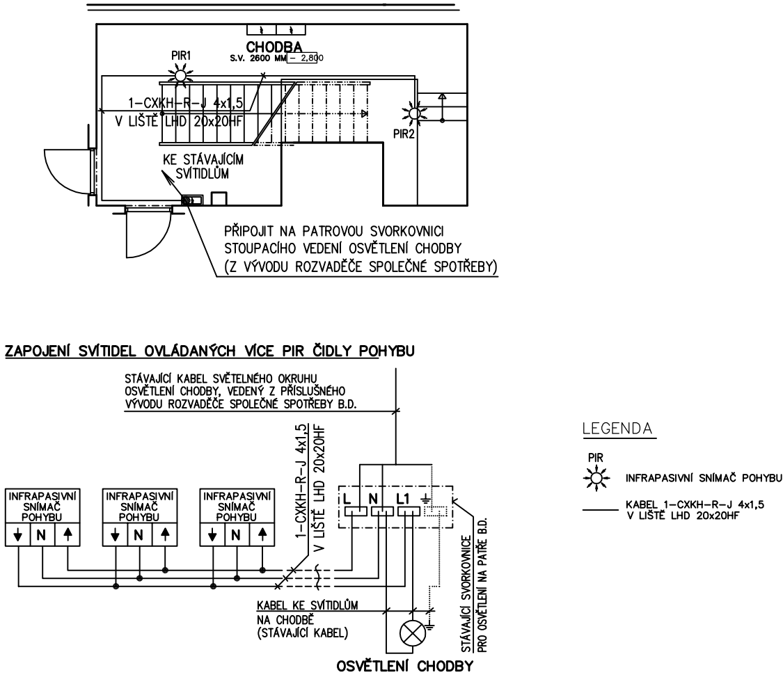
PŮDORYS 1.PP
