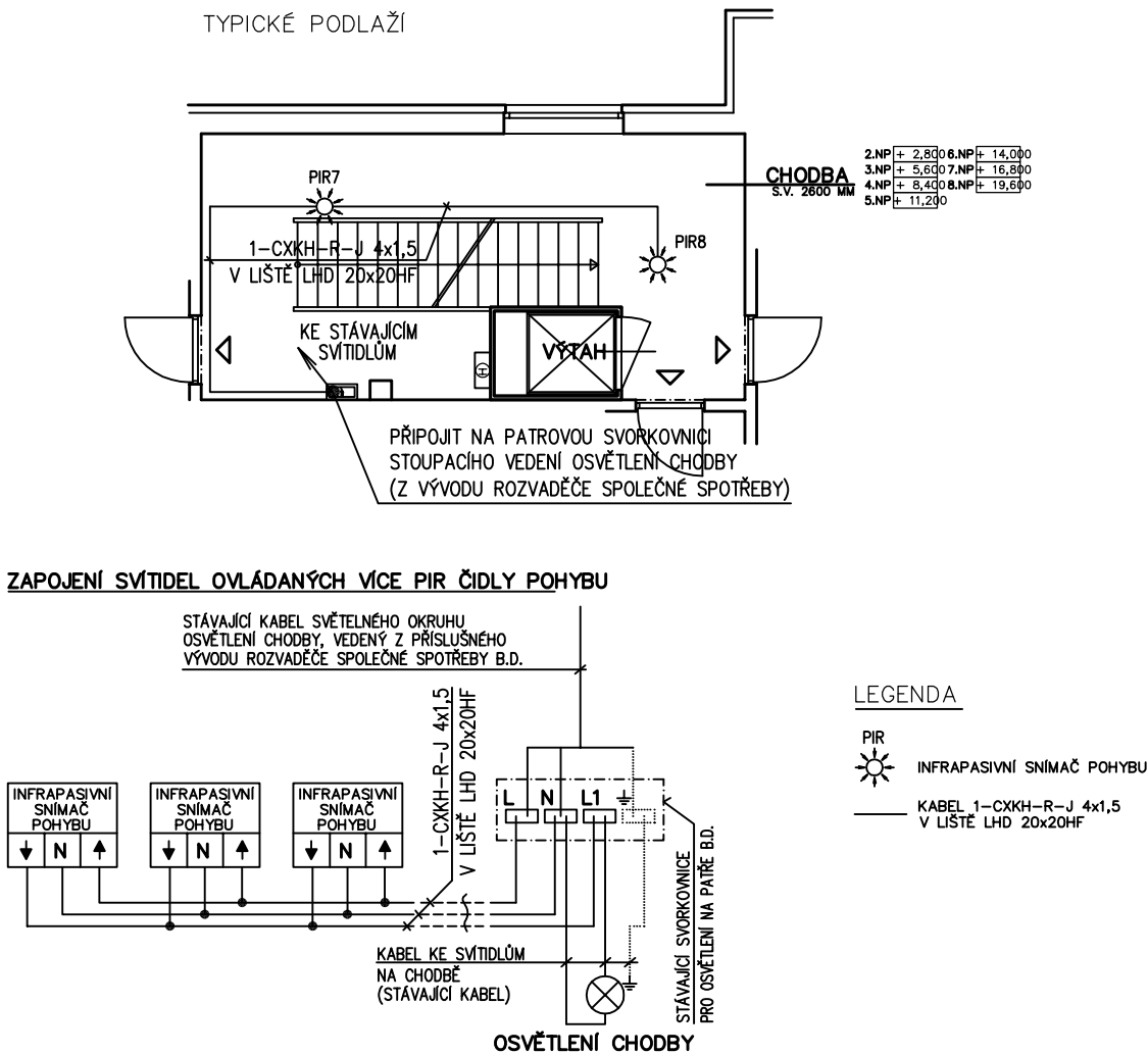
PŮDORYS 2.– 8.NP
